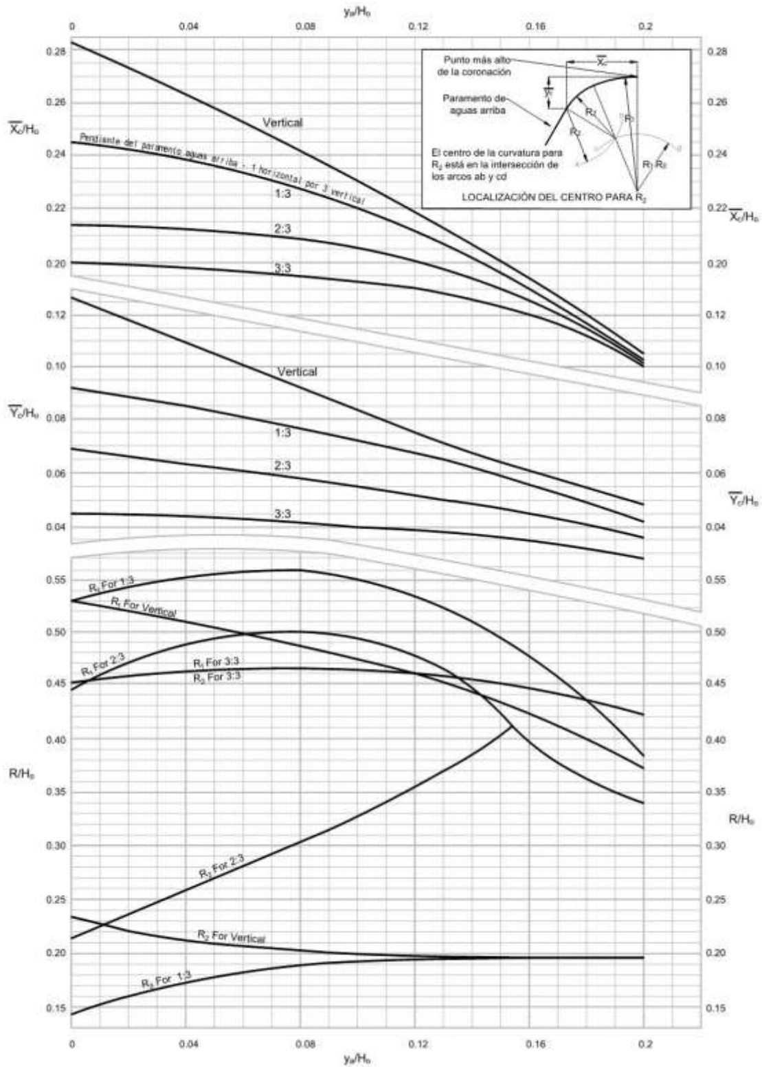
Ilustración 20 Parámetros para la curva de coronación aguas arriba Fuente: (Sotelo Ávila, Diseño hidráulico de estructuras, 1994)
