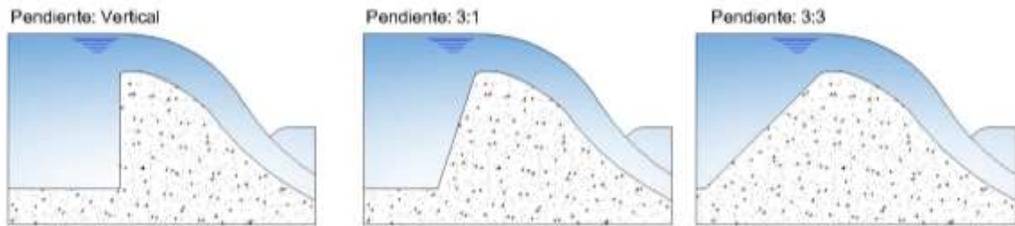
Ilustración 15 Esquemas de paramentos con diferentes pendientes
