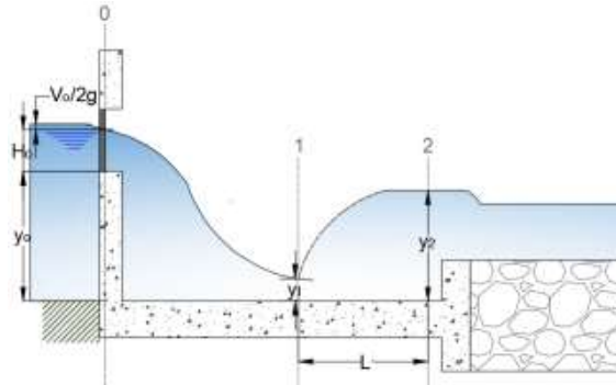
Ilustración 23 Resalto hidráulico
