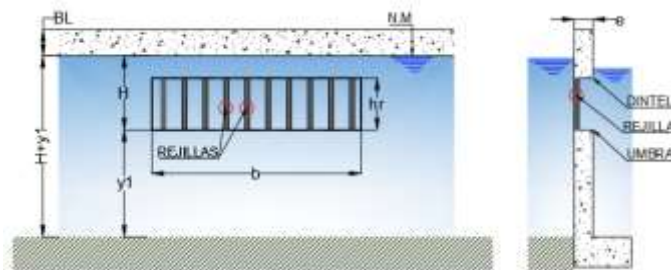
Ilustración 10 Rejilla lateral, trabaja como orificio
