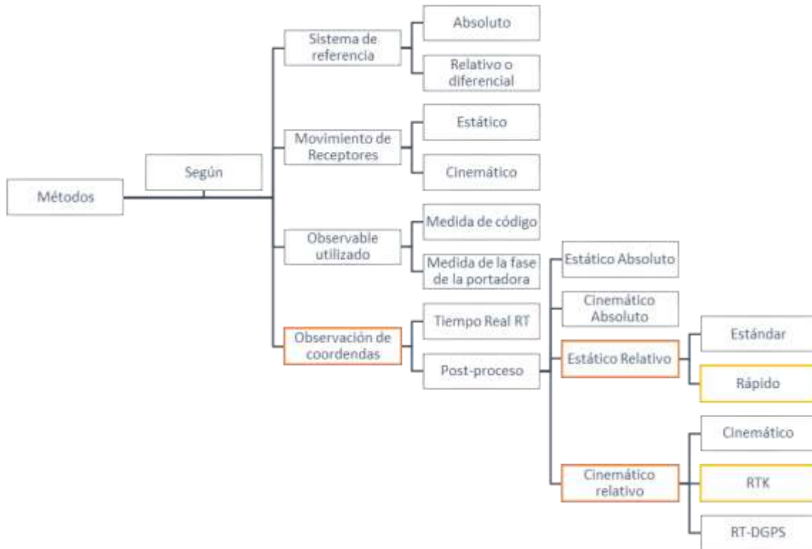
Ilustración 32 Métodos de observación o posicionamiento GPS
