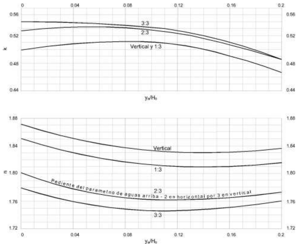
Ilustración 19 Coeficientes que definen el perfil de vertedero Fuente: (Sotelo Ávila, Diseño hidráulico de estructuras, 1994)
