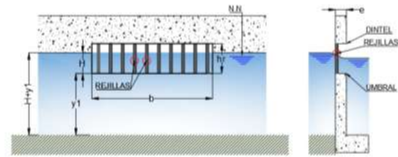
Ilustración 9 Rejilla lateral que trabaja como vertedero
