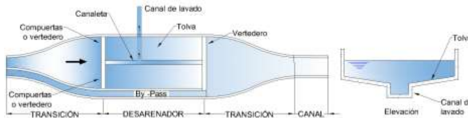
Ilustración 27 Posición y elementos de desarenador de una cámara
