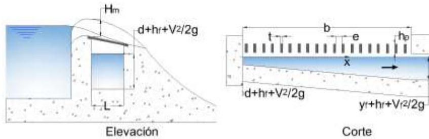
Ilustración 22 Elevación y corte de la rejilla de fondo
