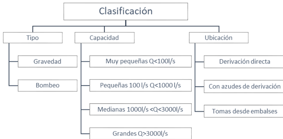
Ilustración 8 Clasificación de captaciones
