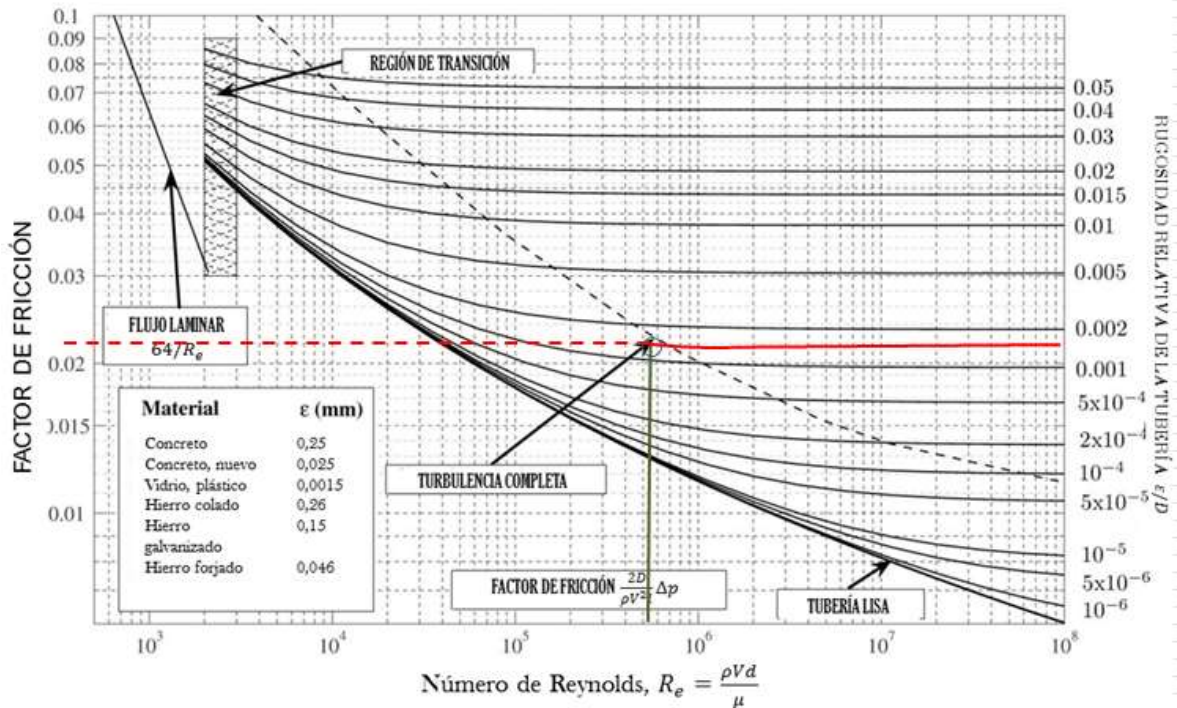
DIAGRAMA DE MOODY
