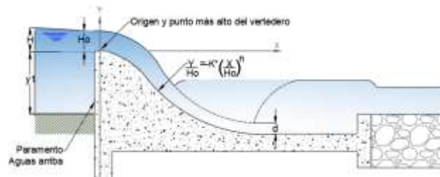
Ilustración 13 Azud
