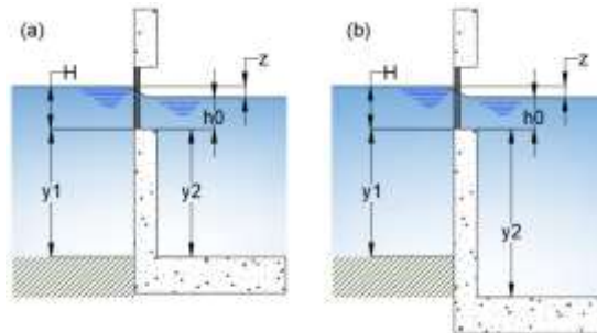
Ilustración 11 Esquema de vertedero sumergido: (a) diseño 1, (b) diseño 2
