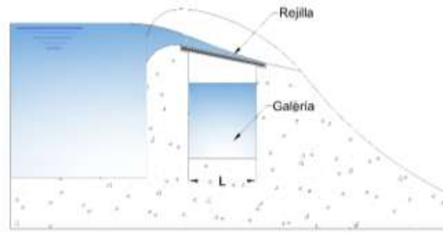
Ilustración 21 Esquema de rejilla de fondo
