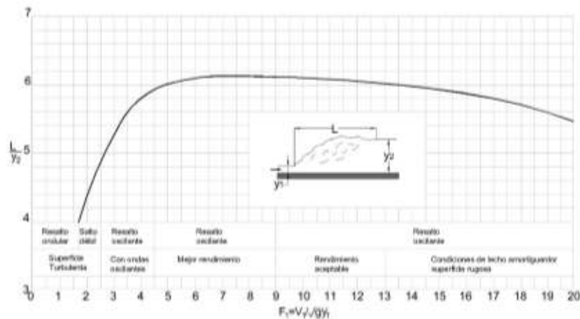
Ilustración 24 Longitud de resalto hidráulico por USBR (United States Bureau of Reclamation)
