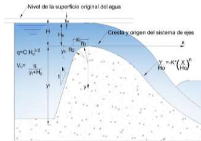
Ilustración 18 Elementos de los perfiles de cimacio con la forma de lámina vertiente
