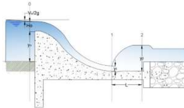
Ilustración 26 Resalto hidráulico al pie del Azud
