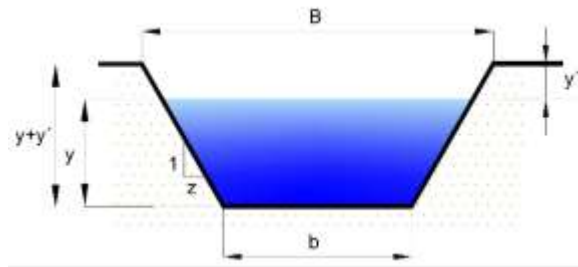
Ilustración 31 Diagrama general de un canal trapecoidal
