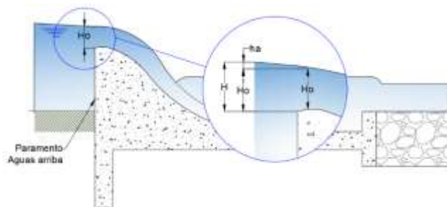
Ilustración 17 Esquema de la carga de diseño
