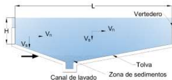
Ilustración 29 Corte del desarenador
