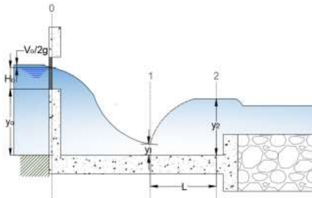
Ilustración 25 Resalto hidráulico en el desripiador
