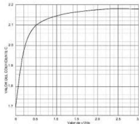
Ilustración 14 Coeficiente de desagüe de un vertedero con paramento vertical
