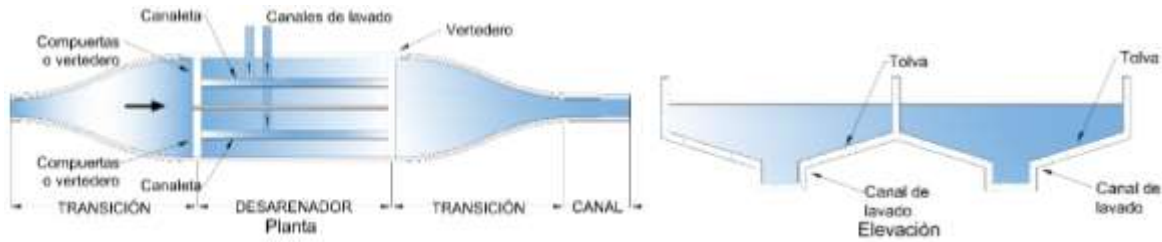
Ilustración 28 Esquema de desarenador de doble cámara
