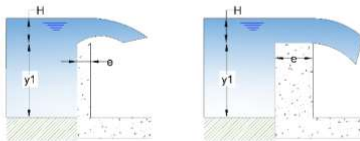
Ilustración 12 Vertedero de cresta delgada y vertederos de cresta gruesa
